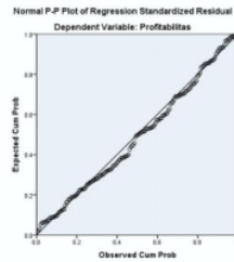
78 Gambar 2. Grafik Normal Plot (setelah outlier)
